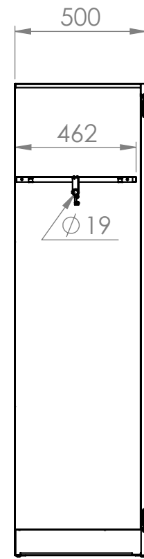
SECTION D-D
