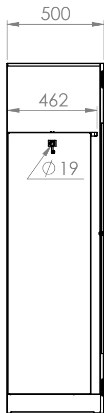
SECTION D-D
