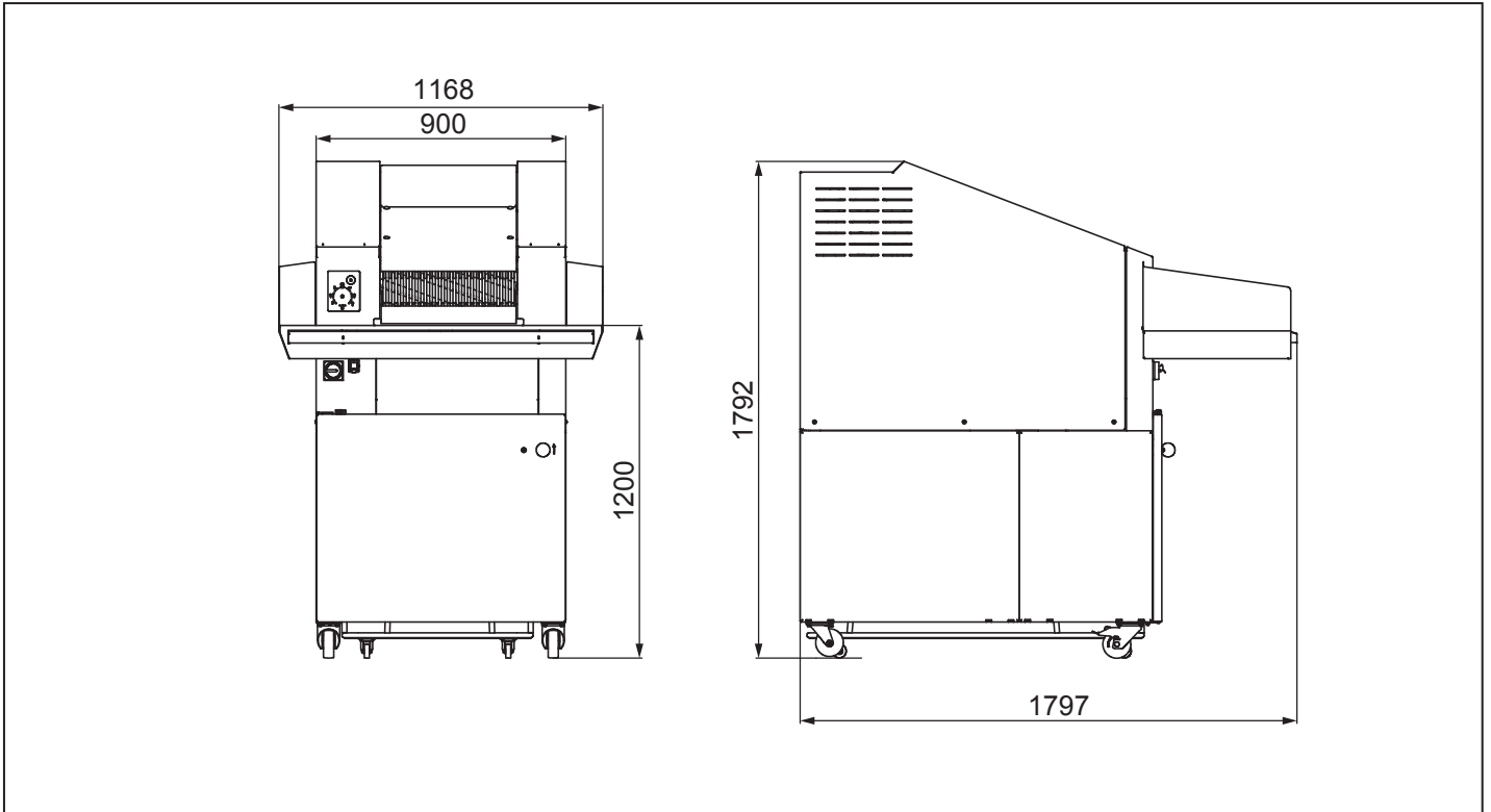
Maße HSM FA 500.3
