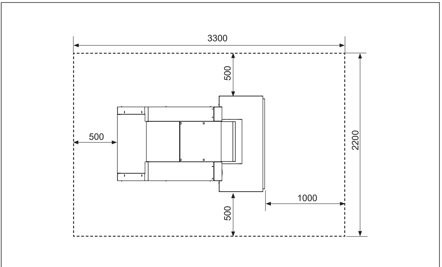
Platzbedarf für Betrieb und Instandhaltung
