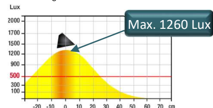
Lichtverteilung Seitenansicht bei 35 cm Abstand
