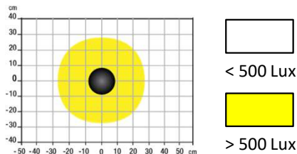
Lichtverteilung Seitenansicht bei 35 cm Abstand
