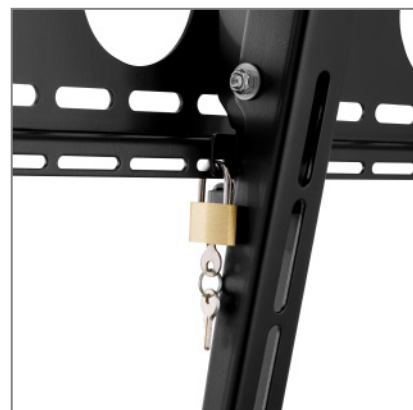
Flacher Wandabstand von nur 65 mm, Schlossfunktion
