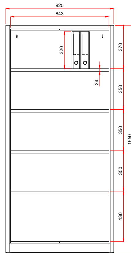
Frontansicht - ohne Türen
